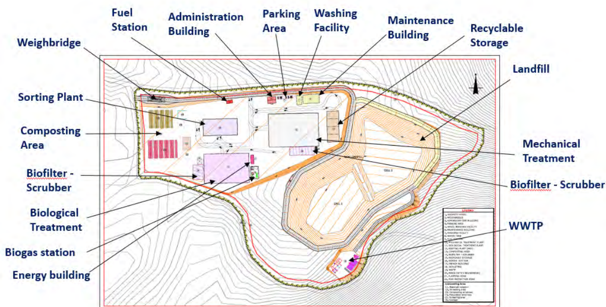
Слика 2: Прелиминарен општ распоред на Центарот за управување со отпад
